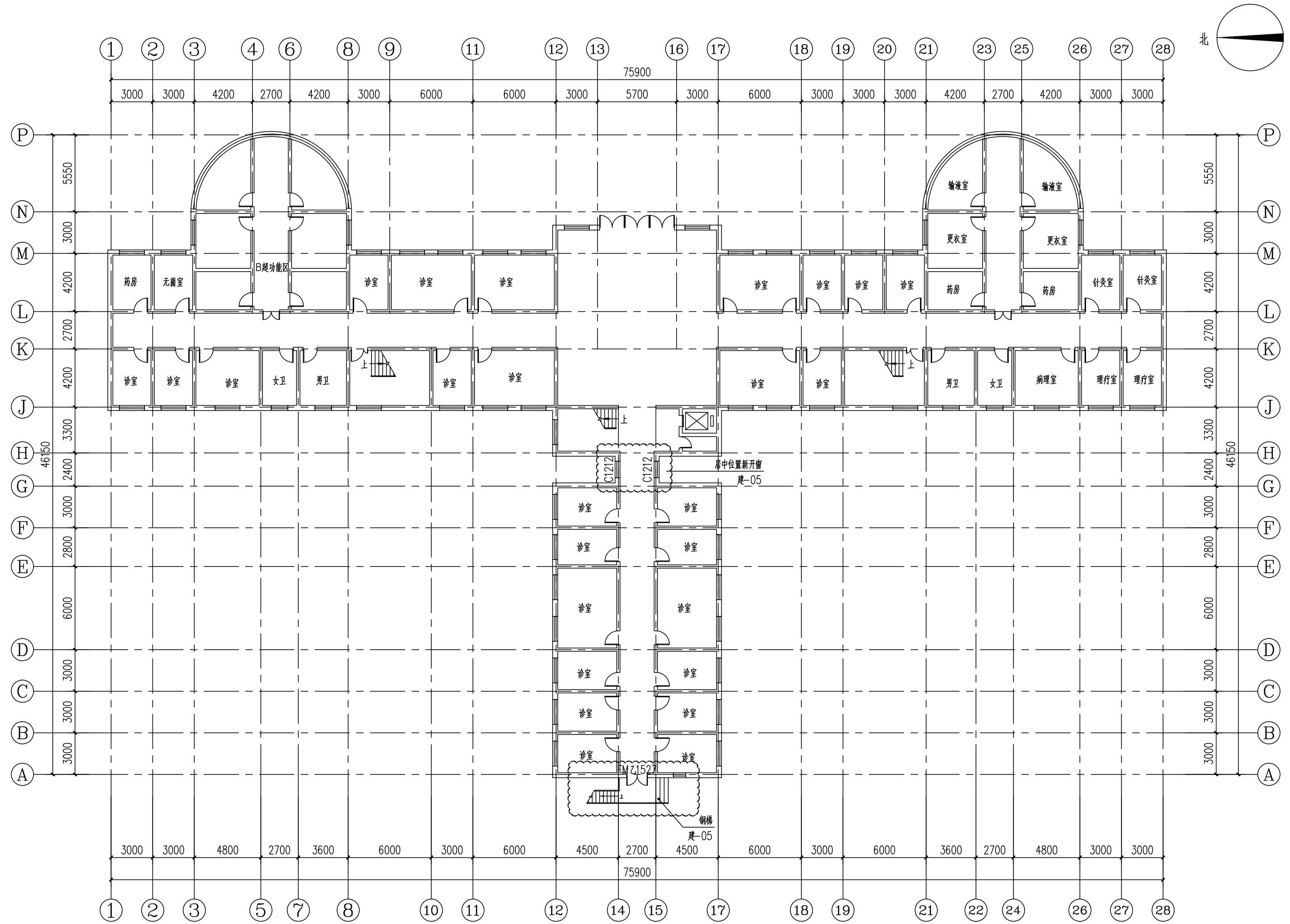
首层平面图 1:200
