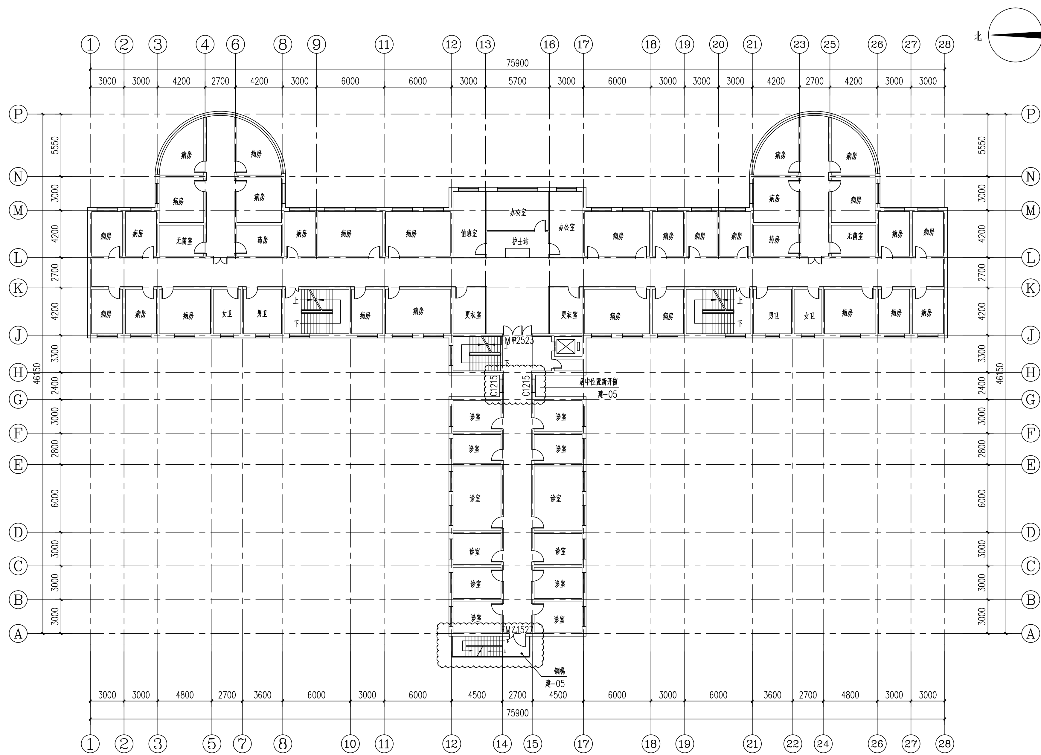
二层平面图 1:200
