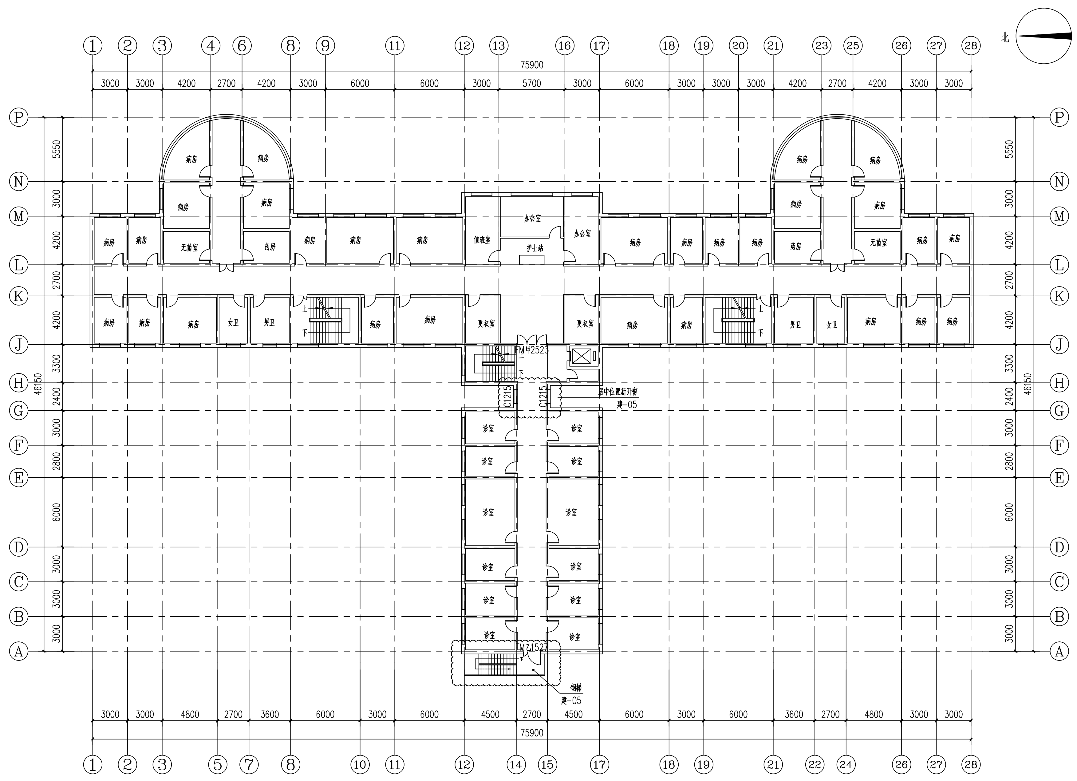
三层平面图 1:200
